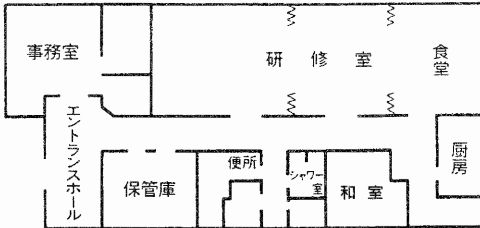
管理棟平面図
